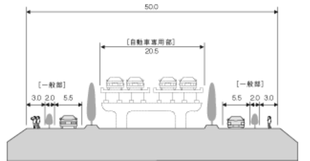
東埼玉道路の一般部と自動車専用部 (単位:m) ※国土交通省北首都国道事務所資料より
